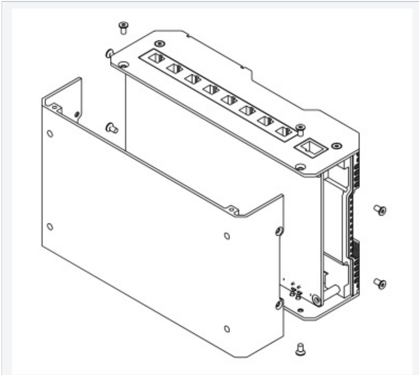
图 打开底盖
