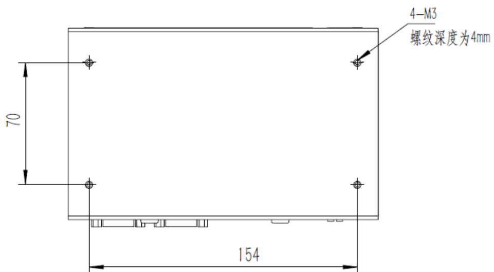
安装孔位图2 Mounting Hole(Unit:mm)
