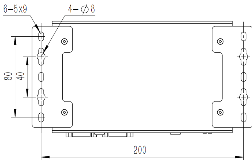
安装孔位图2 Mounting Hole(Unit:mm)
