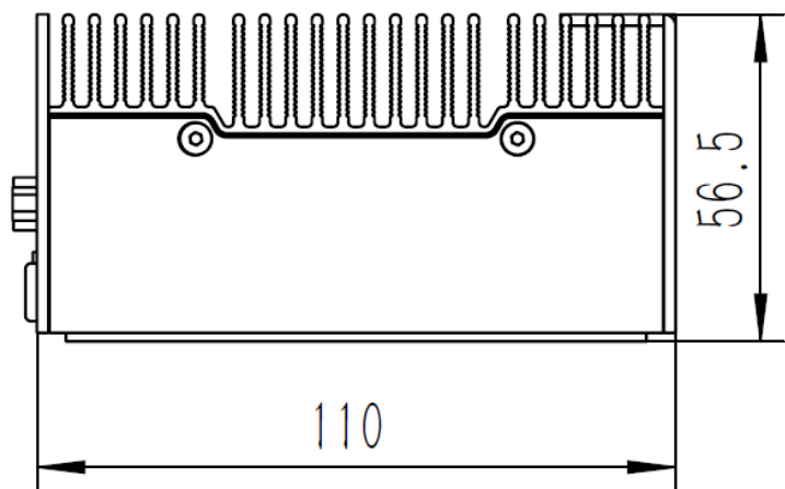
安装孔位图1 Mounting Hole(Unit:mm)
