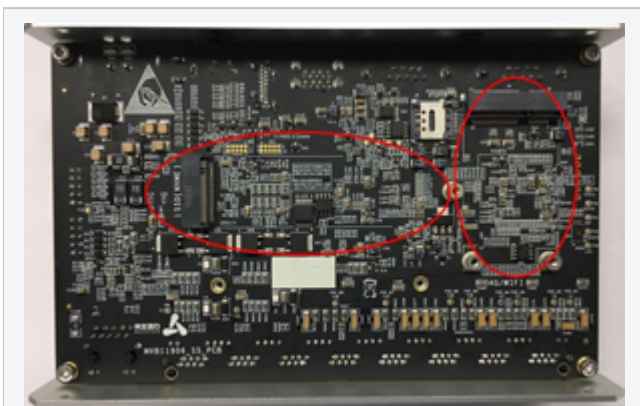
图 可扩展接口位置图
