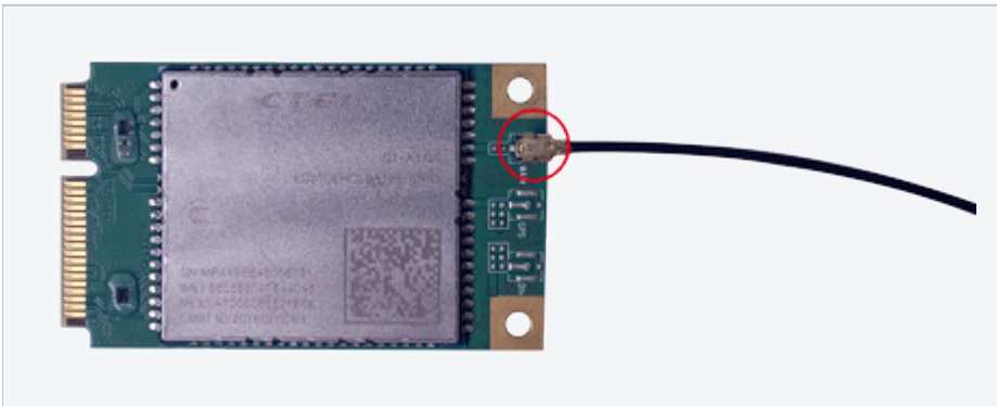
图 天线安装示意图1
