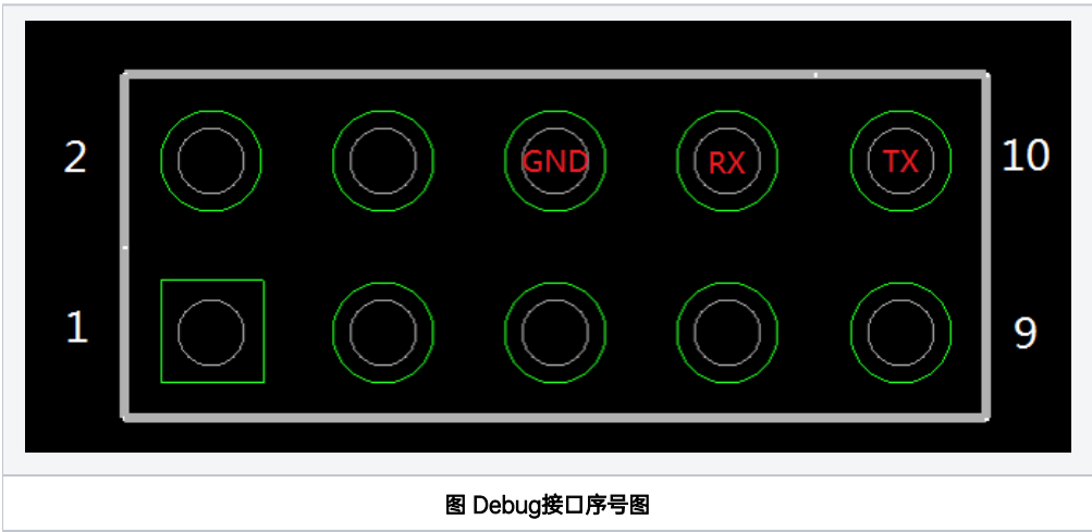
图 Debug接口位置
